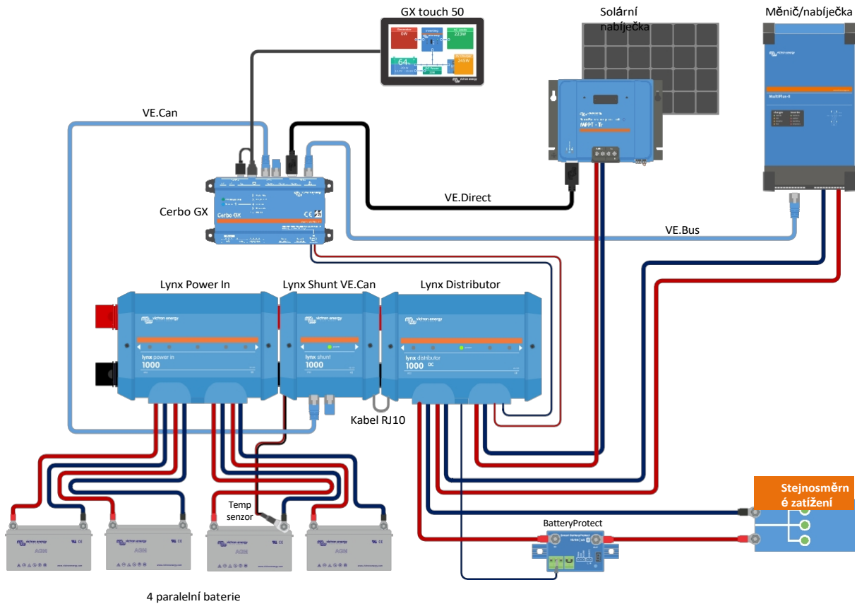
4 paralelní baterie
